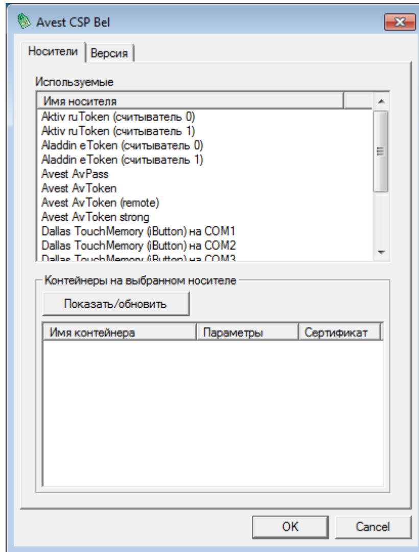
Рисунок 7 - Закладка «Носители»
