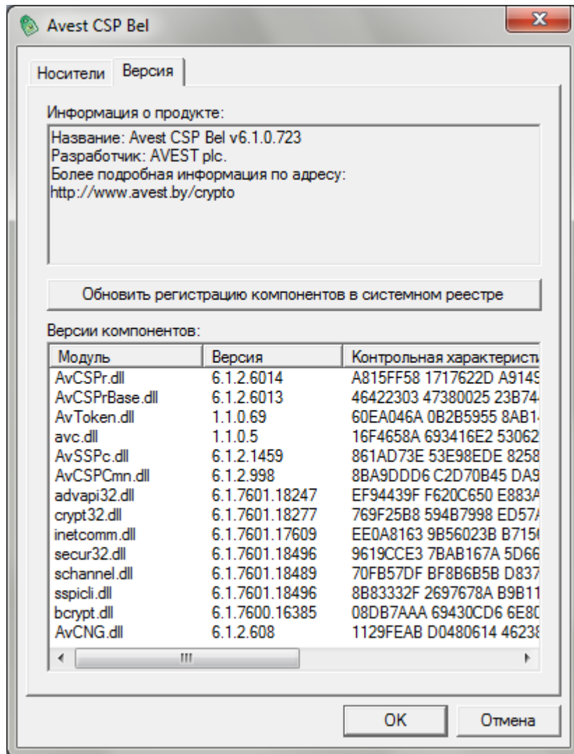
Рисунок 14 - Закладка «Версия»
