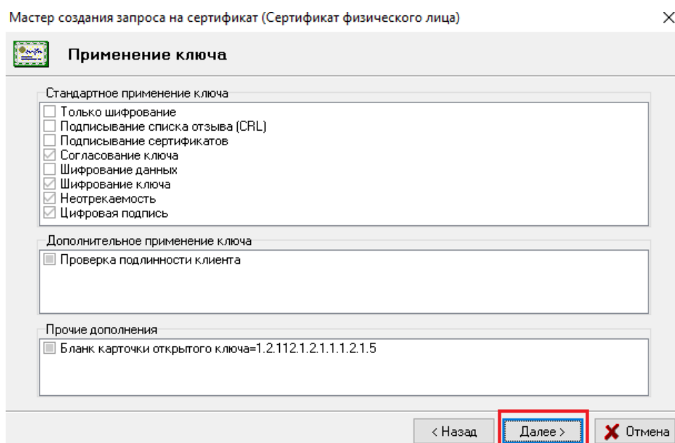
Рисунок 8 – Создание запроса (применение ключа)
